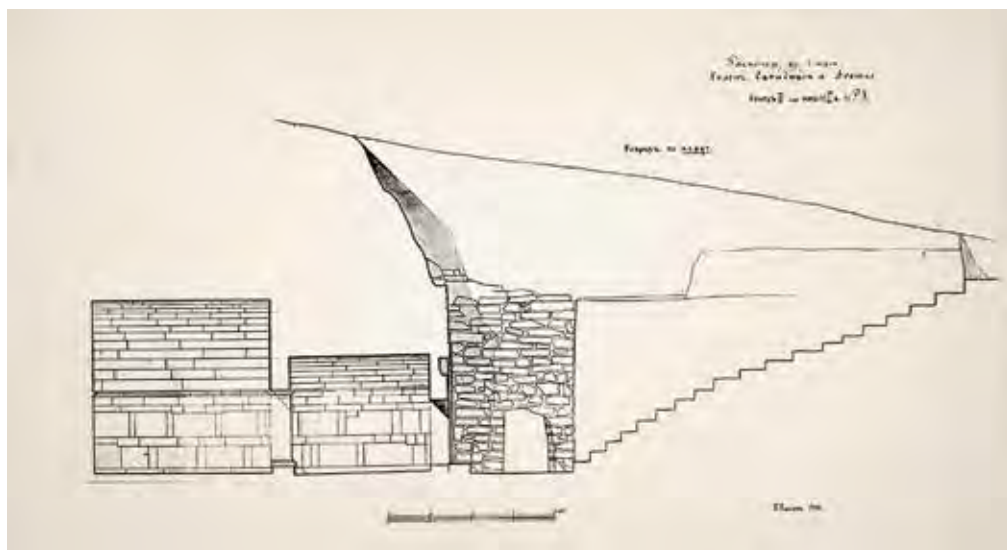
Ольвия. Склеп Еврисивия и Ареты (конец II — начало III в. н. э.). Чертеж К. К. Романова, 1908 г. (ФО. Отп. O.1767-49)
