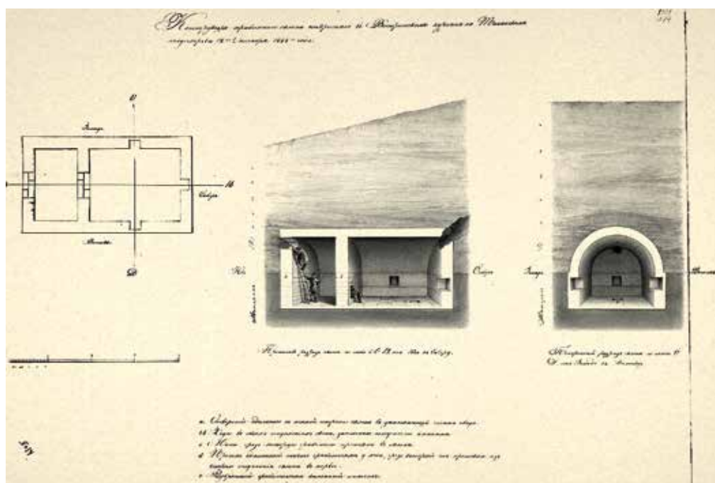
Ограбленный склеп Васюринской горы, открытый 12 октября 1868 г. (РО. Р-1. Оп. 1. Д. 565. Л. 8)
