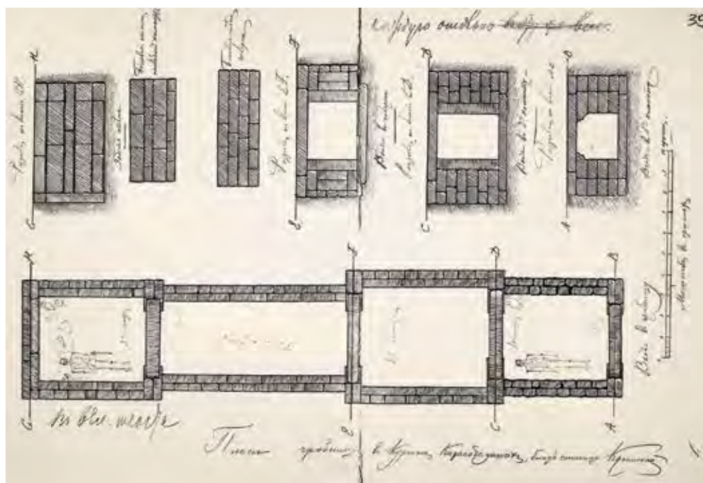
План гробницы кургана Карагодеуаш. Раскопки Е. Д. Фелицына (РО. Ф. 1. Оп. 1-1886 г. Д. 16. Л. 35 об. — 35а)
