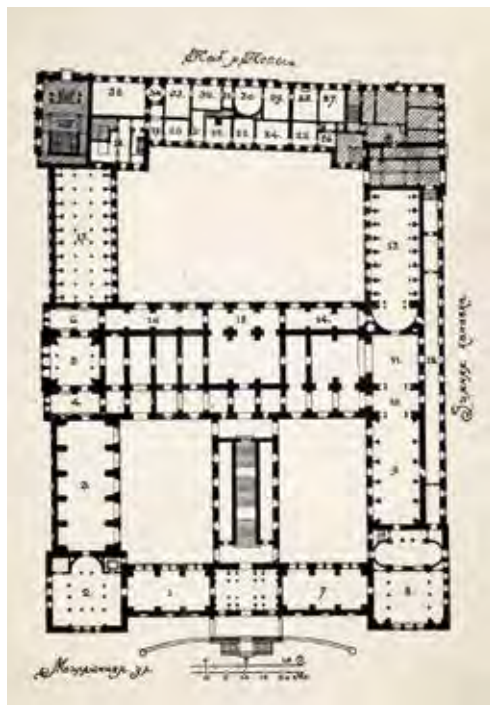
План Нового Эрмитажа: помещения Императорской археологической комиссии после переезда 1882 г. располагались на углу Зимней канавки и Миллионной улицы (по: Макаренко 1916)
